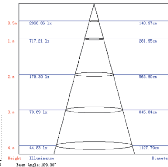
ULO-ZL60-25W/NW WHITE
